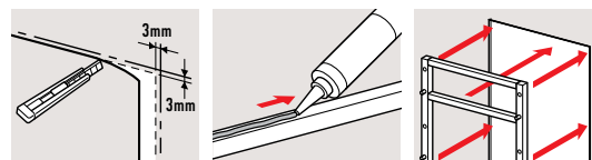
① 切り込みを入れてクロスをはがす。 ② 受け枠に専用接着剤を塗る。 ③ 受け枠をクロスをはがした部分に貼付ける。
